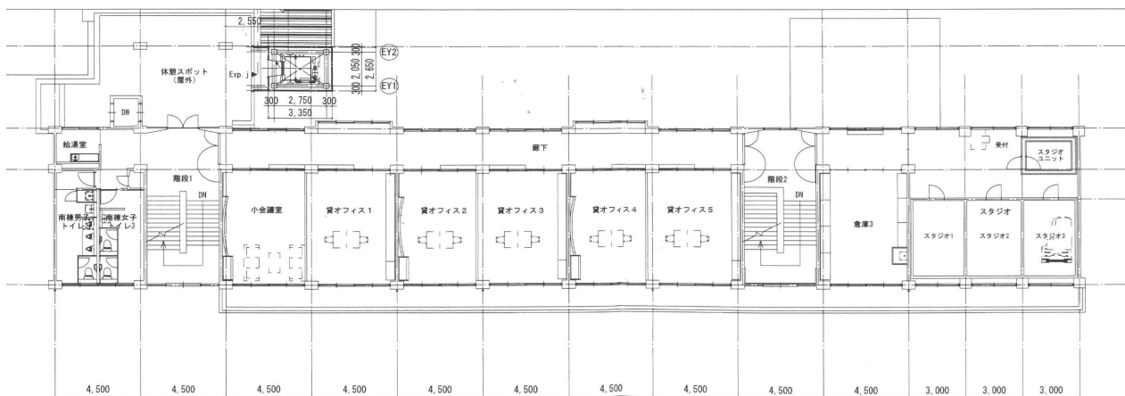
《南棟3階平面図》
